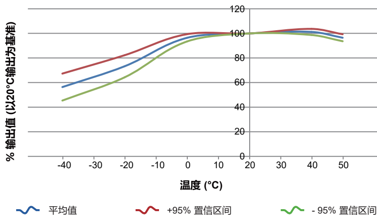
盛密科技WC Air Quality传感器温度性能
